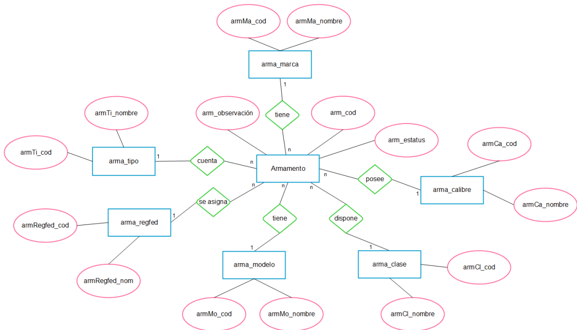
Figura 3.20 Modelo entidad-relación del inventario de armamento en la base de datos edofuerza (Elaboración propia, 2018)
