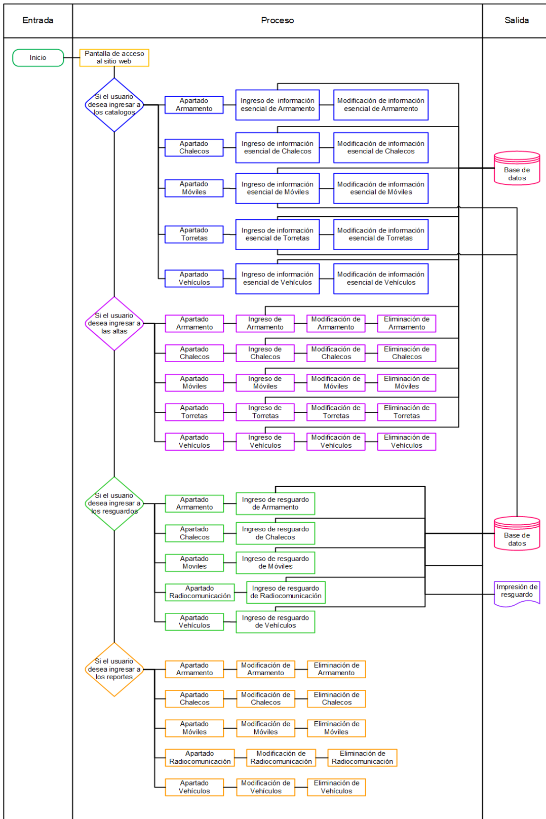
Figura 3.19 Diagrama HIPO (Elaboración propia, 2018)
