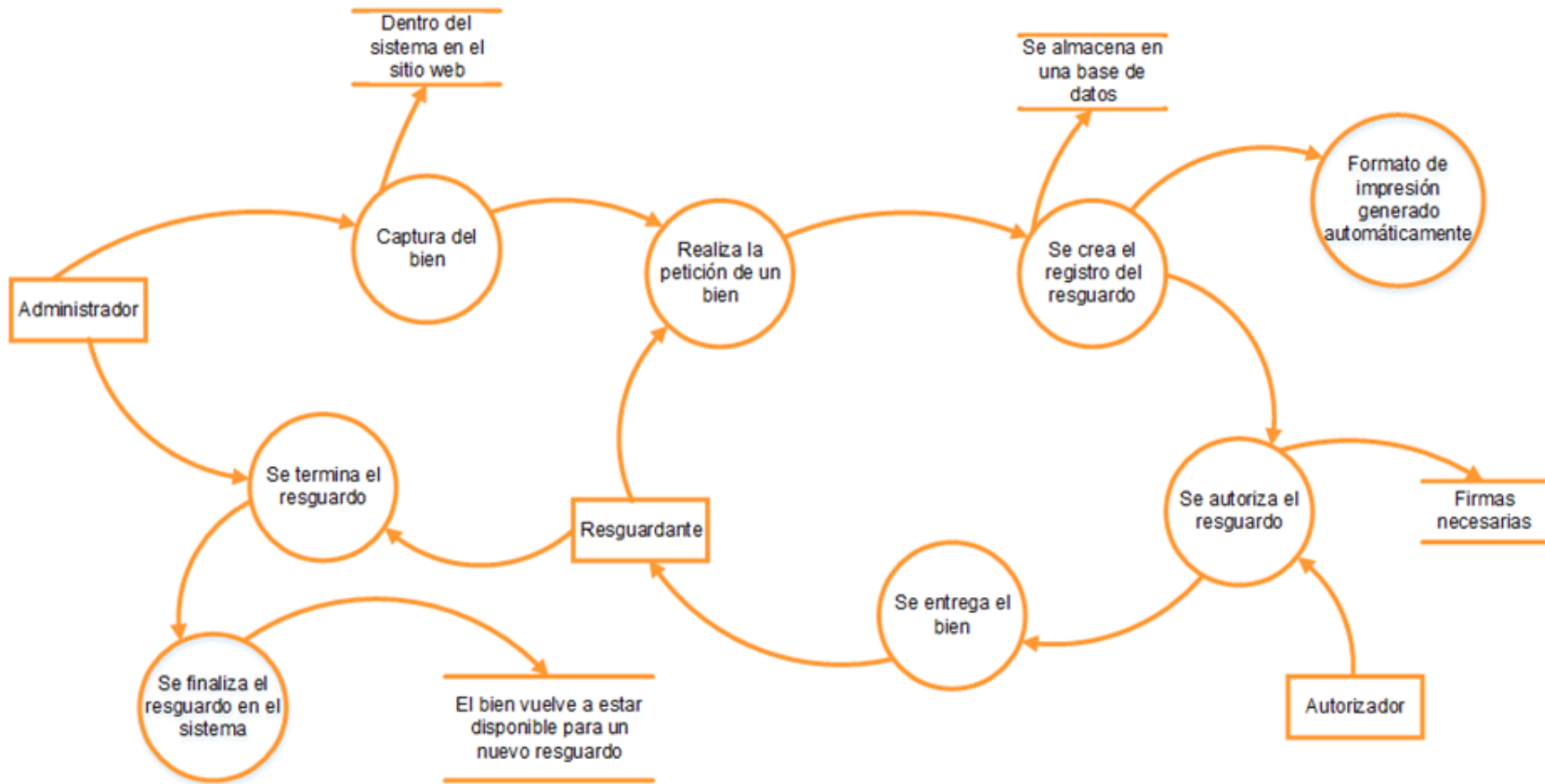
Figura 3.10 Diagrama de flujo de datos del sistema futuro Fase 2 (Elaboración propia, 2018)
