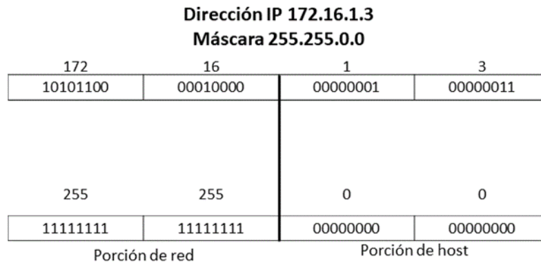
Figura 2.11 Ejemplo de dirección IPv4 (Ariganello, 2016)
