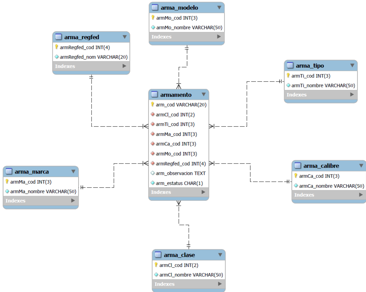
Figura 3.22 Modelo relacional del inventario de armamento en la base de datos edofuerza (Elaboración propia, 2018)
