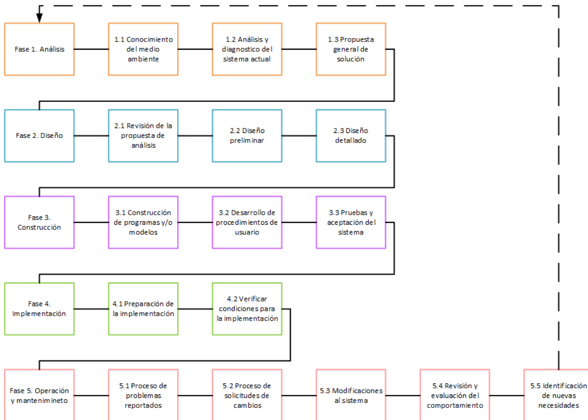
Figura 2.12 Metodología para el desarrollo del sistema de información basado en computadoras
