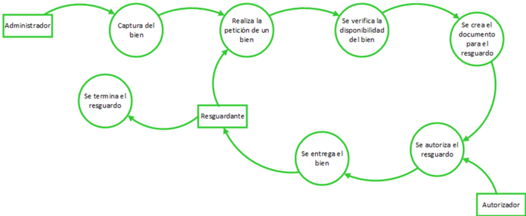
Figura 3.6 Diagrama de flujo de datos del sistema actual Fase 1 (Elaboración propia, 2018)
