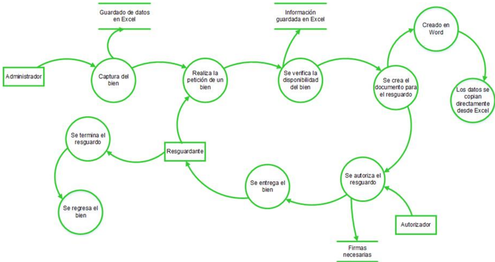
Figura 3.7 Diagrama de flujo de datos del sistema actual Fase 2 (Elaboración propia, 2018)
