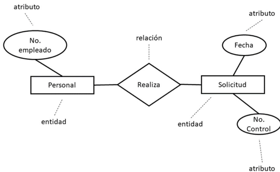
Figura 2.4 Ejemplo del Modelo Entidad-Relación (Elaboración propia, 2018)
