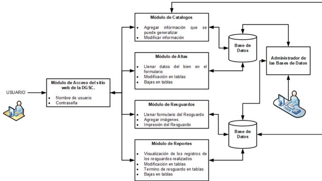
Figura 3.12 Arquitectura del sistema (Elaboración propia, 2018)
