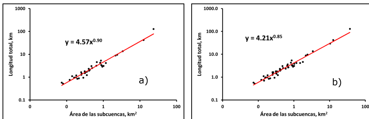
Figura 4. Gráficos para la estimación del parámetro \varepsilon , empleado en cálculo de la dimensión fractal de la red: a) río San Cristóbal, b) río Santa Cruz. El eje de las ordenadas representa la longitud total de todas las corrientes que caen dentro de una subcuenca.
