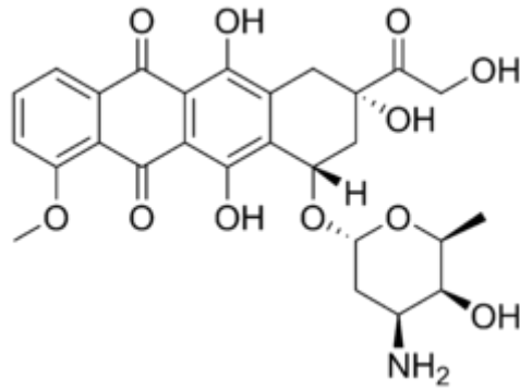
Figura 1.1 Doxorubicina.
